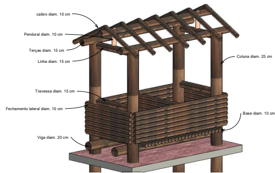
5 Estrutura Telhado
