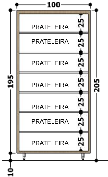
VISTA INTERNA – ARMÁRIO COM 2 PORTAS.
