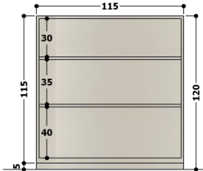
VISTA FRONTAL – ARMÁRIO COM PRATELEIRAS.
