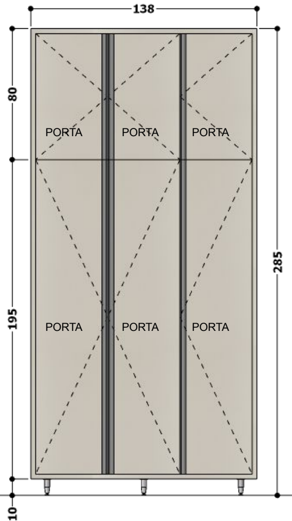
VISTA FRONTAL – ARMÁRIO COM PORTAS PISO A TETO.
