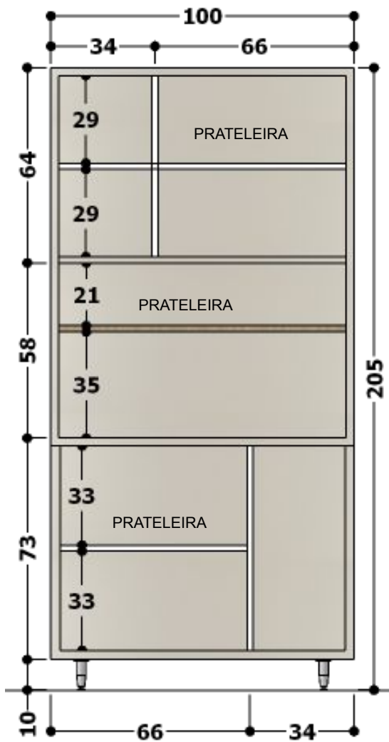
VISTA INTERNA – GABINETE COM PORTAS E GAVETAS.
