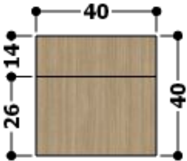
VISTA SUPERIOR (PLANTA) – VISTA FRONTAL – GABINETE COM PORTA E GAVETAS.
