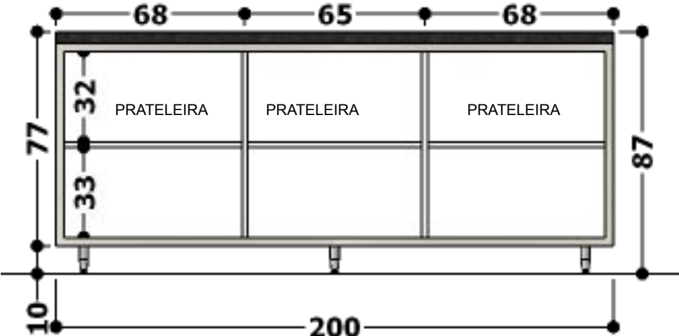
VISTA INTERNO – GABINETE COM PORTAS.
