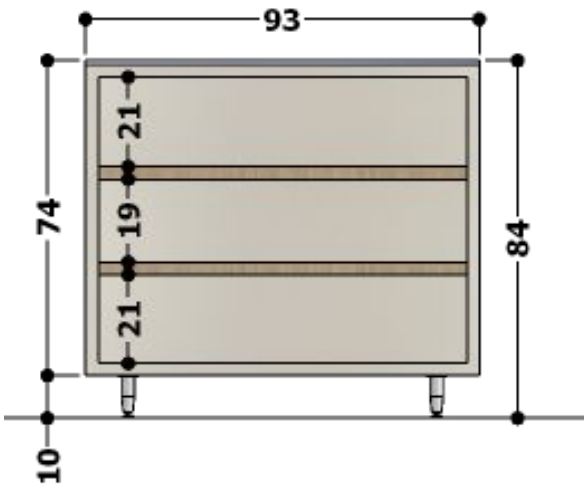
VISTA FRONTAL – APARADOR COM TAMPO DE VIDRO.
