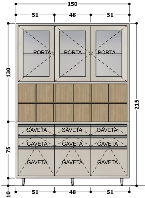
VISTA FRONTAL – ARMÁRIO COM PORTAS E GAVETAS.
