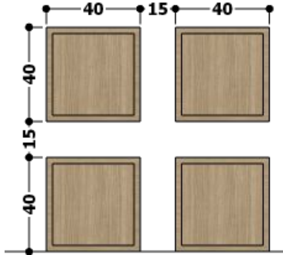
VISTA FRONTAL – NICHOS.
