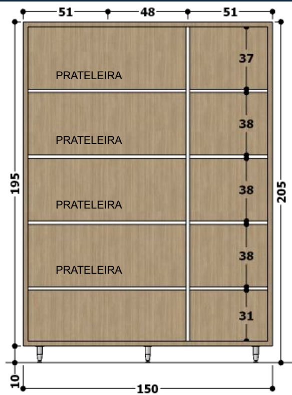
VISTA INTERNA – ARMÁRIO COM PORTAS.
