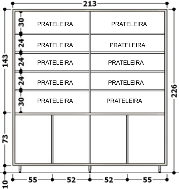
VISTA INTERNA – ARMÁRIO COM PORTAS E GAVETAS.
