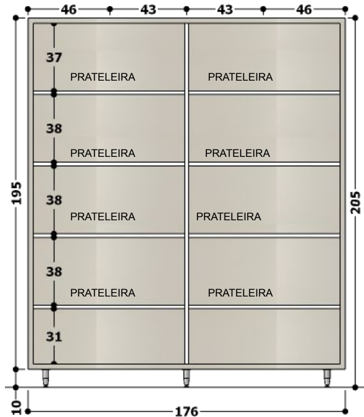
VISTA INTERNA – ARMÁRIO COM PORTAS.
