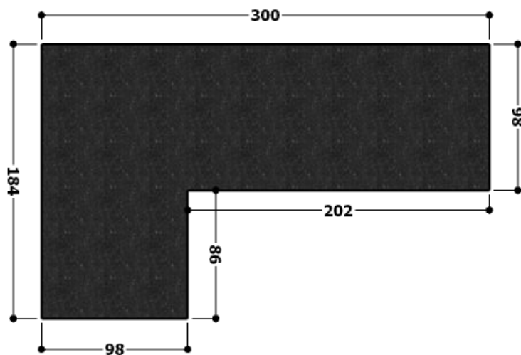
VISTA SUPERIOR (PLANTA) – GABINETE EM L.
