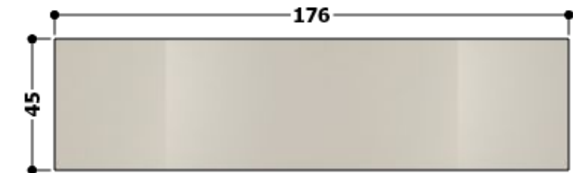
VISTA SUPERIOR (PLANTA) – ARMÁRIO COM PORTAS.
