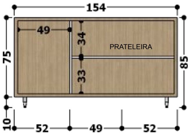
VISTA INTERNA – BANCADA COM PORTAS E LIXEIRA.
