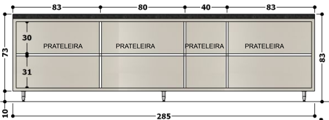
VISTA INTERNA – BALCÃO COM PORTAS.
