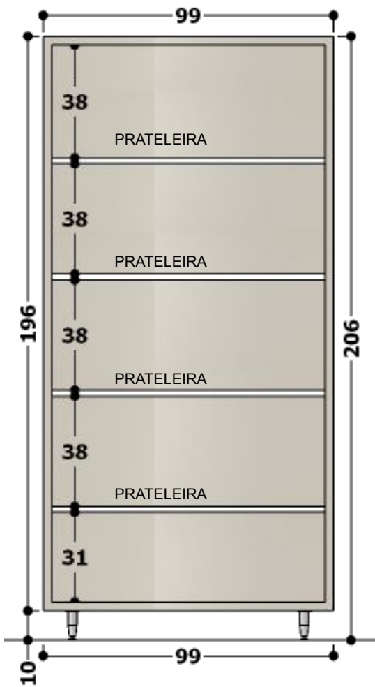
VISTA INTERNA – ARMÁRIO COM PORTAS.
