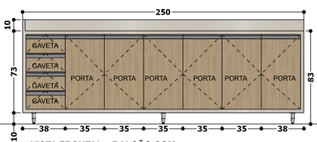
VISTA FRONTAL – BALCÃO COM PORTAS.
