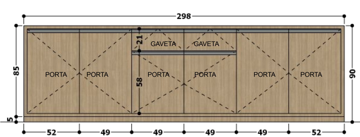
VISTA FRONTAL – BALCÃO COM PORTAS.
