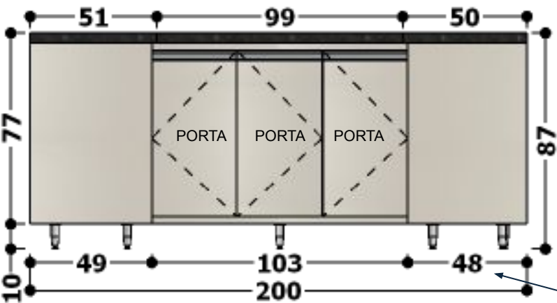
VISTA FRONTAL – GABINETE EM U COM PORTAS.
