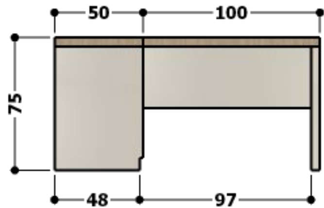
VISTA FRONTAL – MESA EM L COM GAVETAS.
