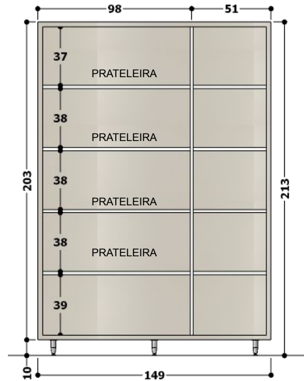
VISTA INTERNO – ARMÁRIO COM PORTAS.
