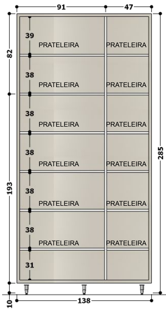
VISTA INTERNA – ARMÁRIO COM PORTAS PISO A TETO.
