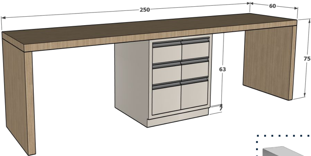
VISTA PERSPECTIVADA – MESA RECEPÇÃO
