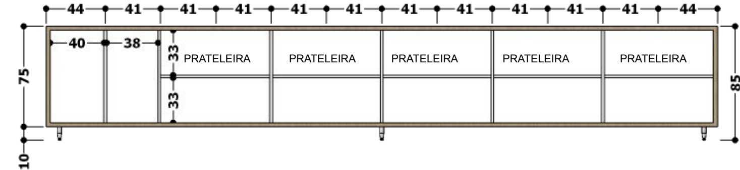
VISTA INTERNA – ARMÁRIO BAIXO COM PORTAS.
