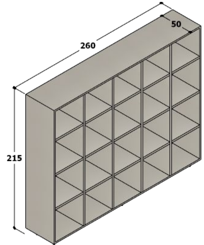
VISTA PERSPECTIVADA – ARMÁRIO DE NICHOS.
