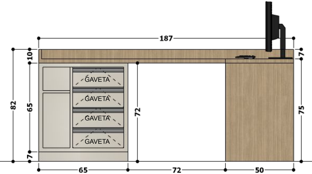
VISTA FRONTAL – MESA EM L COM ARMÁRIO E GAVETAS.
