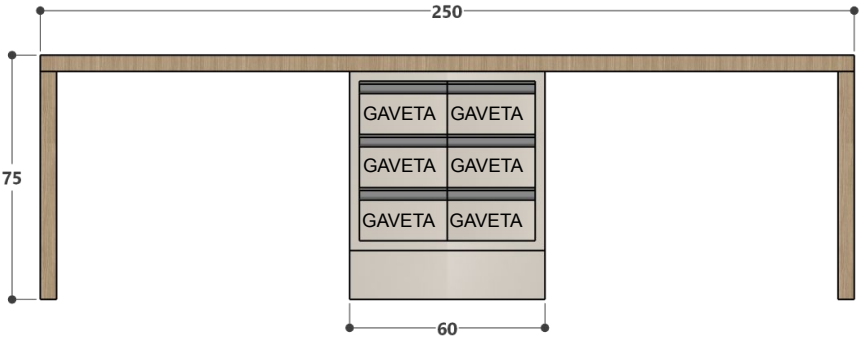
VISTA FRONTAL – MESA RECEPÇÃO
