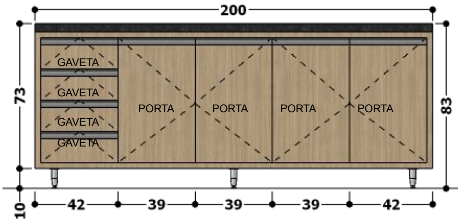
VISTA FRONTAL – GABINETE COM PORTAS E GAVETAS.
