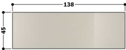
VISTA SUPERIOR (PLANTA) – ARMÁRIO COM PORTAS PISO A TETO.
