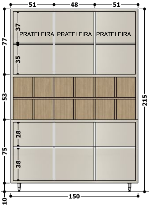
VISTA INTERNA – ARMÁRIO COM PORTAS E GAVETAS.
