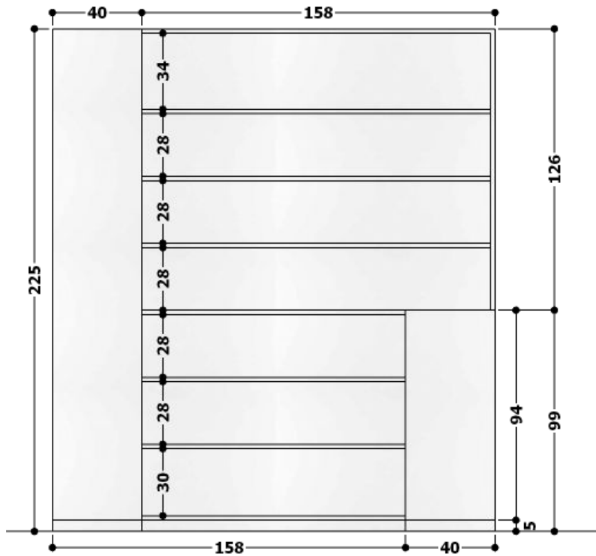
VISTA FRONTAL – ARMÁRIO EM L.
