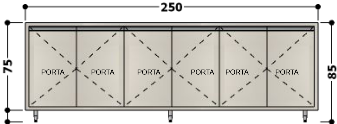
VISTA FRONTAL – BALCÃO COM PORTAS.
