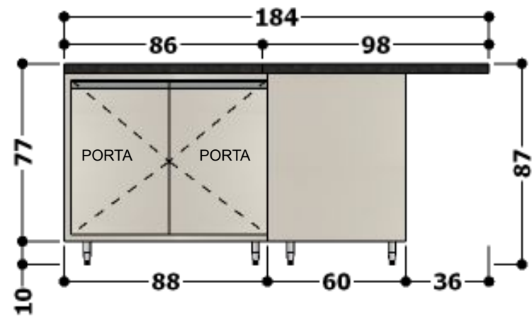
VISTA FRONTAL – GABINETE EM L.
