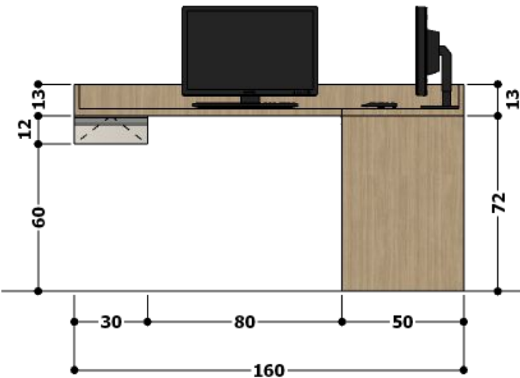
VISTA LATERAL – MESA EM L COM GAVETAS.
