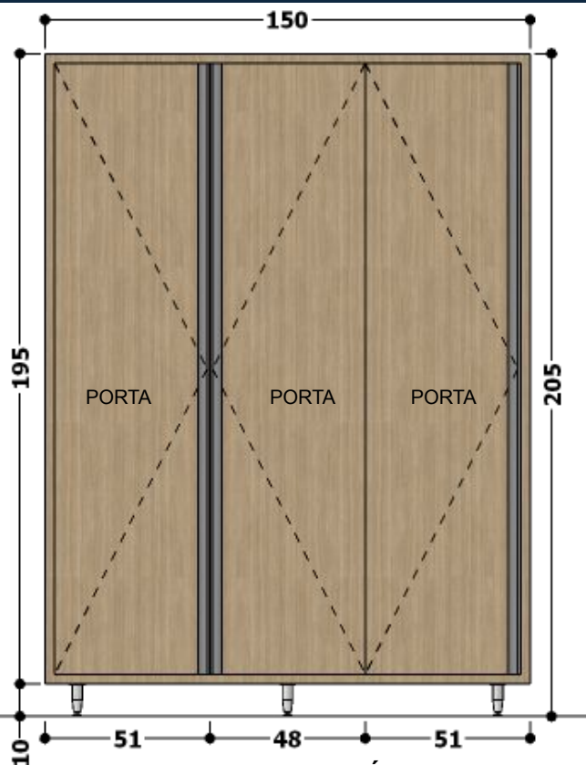
VISTA FRONTAL – ARMÁRIO COM PORTAS.
