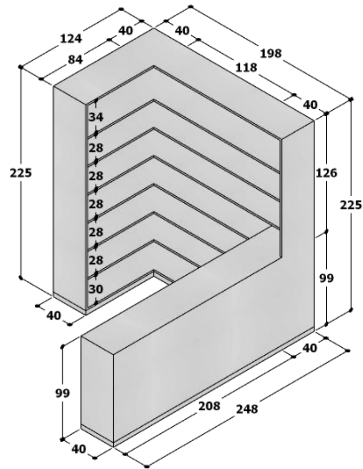
VISTA PERSPECTIVADA – ARMÁRIO EM L.
