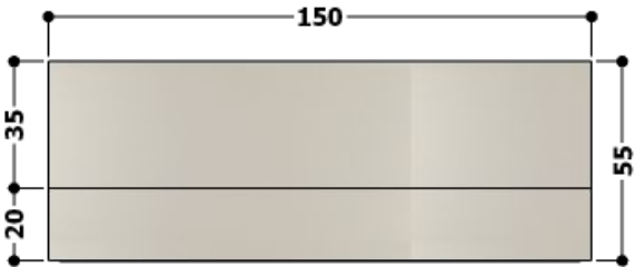
VISTA SUPERIOR (PLANTA) – ARMÁRIO COM PORTAS E GAVETAS.
