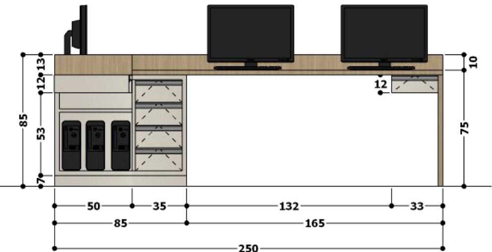
VISTA FRONTAL – MESA EM L COM GAVETAS.
