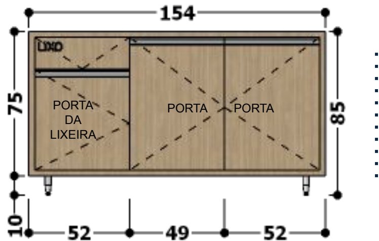
VISTA FRONTAL – BANCADA COM PORTAS E LIXEIRA.
