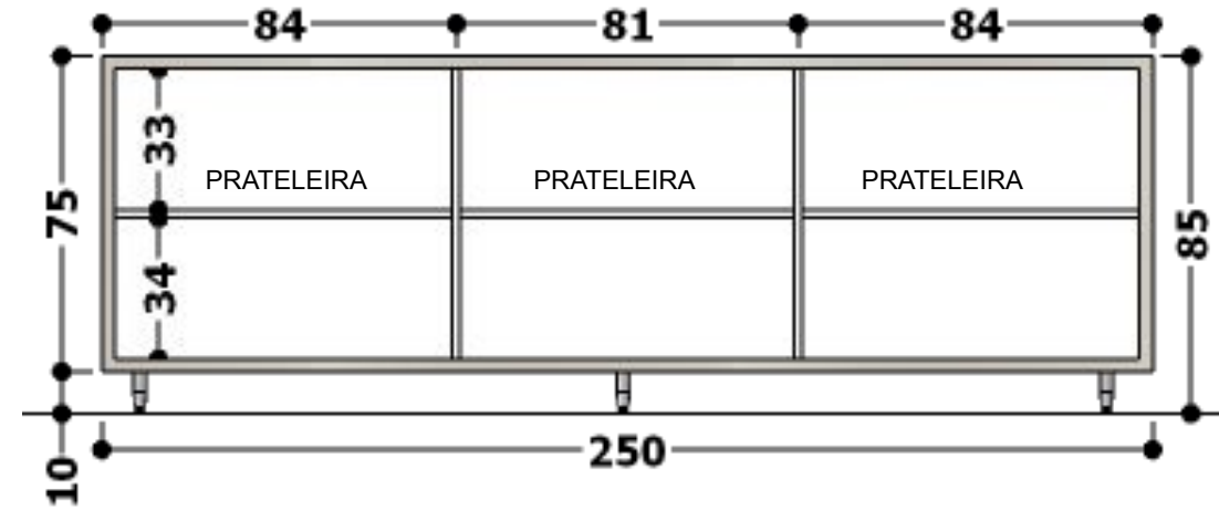
VISTA INTERNA – BALCÃO COM PORTAS.
