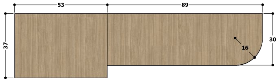
VISTA SUPERIOR (PLANTA) – NICHOPARA MICROONDAS.
