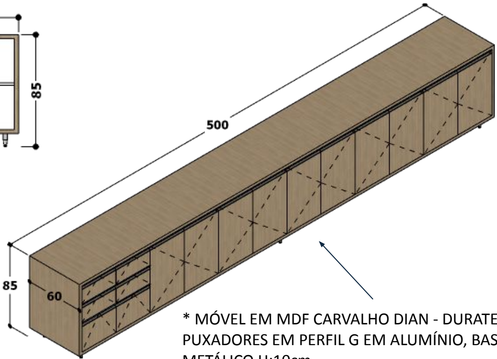
VISTA PERSPECTIVADA – ARMÁRIO BAIXO COM PORTAS.
