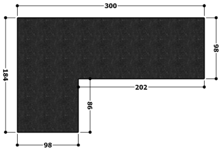
VISTA SUPERIOR (PLANTA) – GABINETE EM L.
