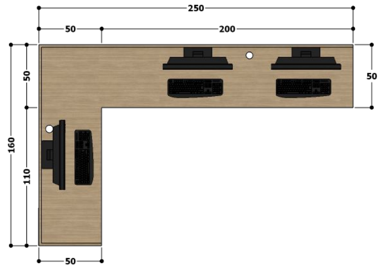
VISTA SUPERIOR (PLANTA) – MESA EM L COM GAVETAS.
