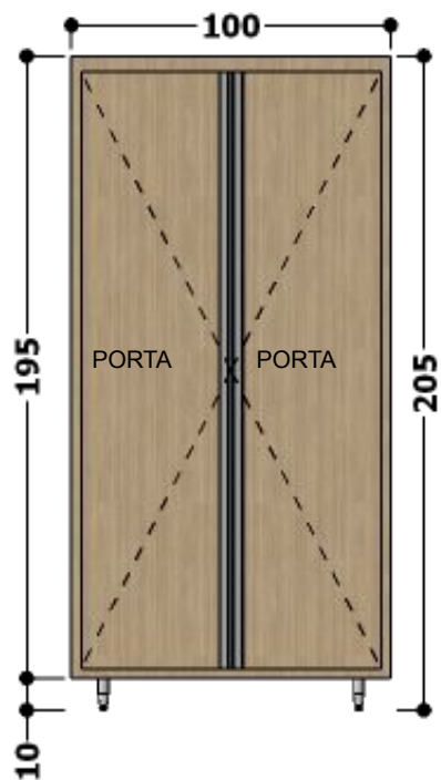
VISTA FRONTAL – ARMÁRIO COM 2 PORTAS.
