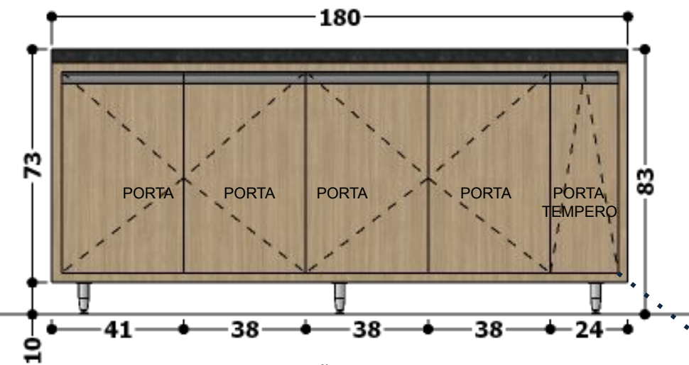
VISTA FRONTAL – BALCÃO COM PORTAS.
