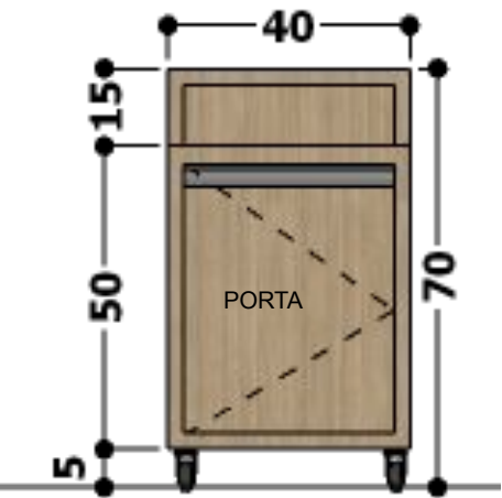
VISTA FRONTAL – MESA DE APOIO COM PORTA E RODÍZIO.
