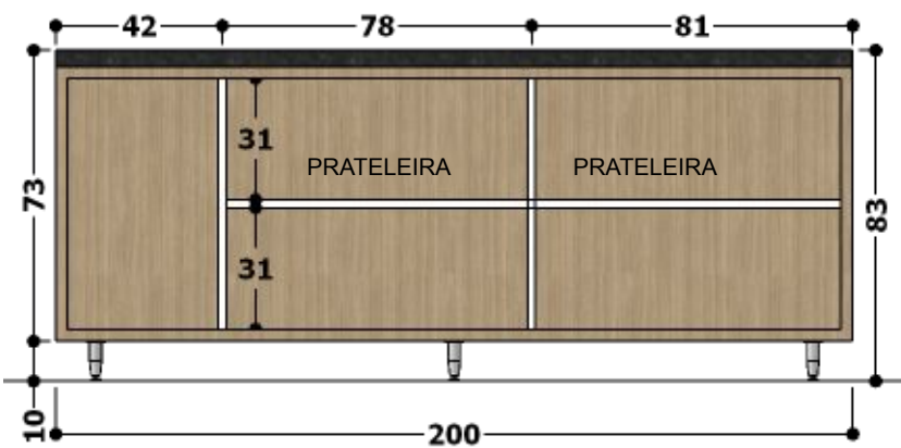
VISTA INTERNA – GABINETE COM PORTAS E GAVETAS.
