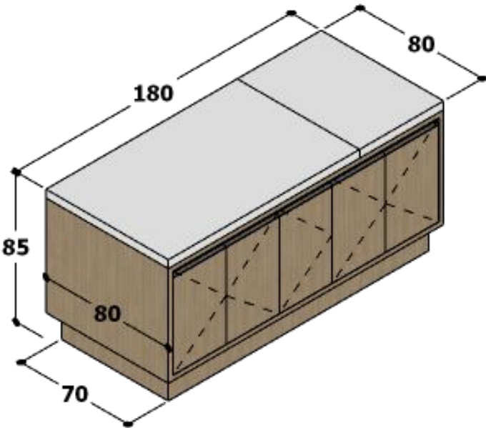
VISTA PERSPECTIVADA DIREITA – MACA COM PORTAS NAS LATERAIS.
