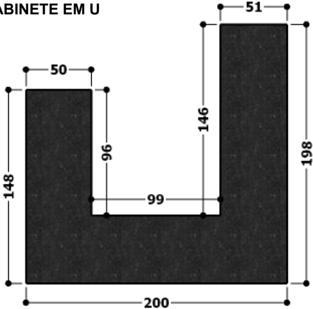
VISTA SUPERIOR (PLANTA) – GABINETE EM U COM PORTAS.
