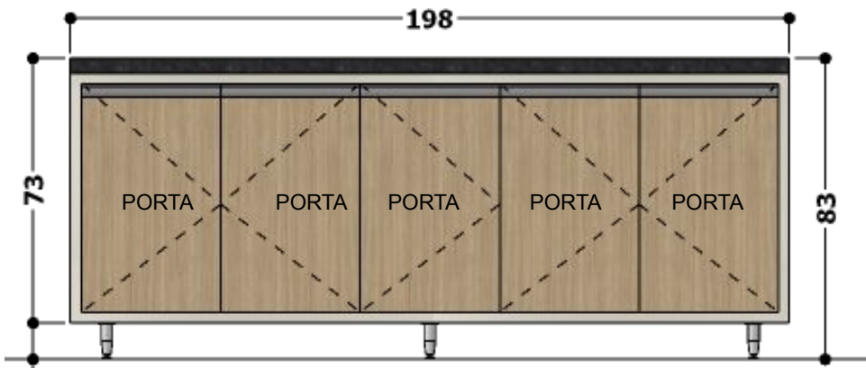
VISTA FRONTAL – GABINETE COM PORTAS.
