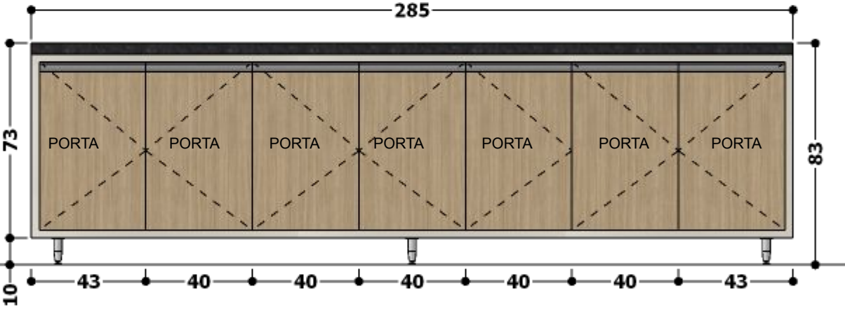
VISTA FRONTAL – BALCÃO COM PORTAS.
