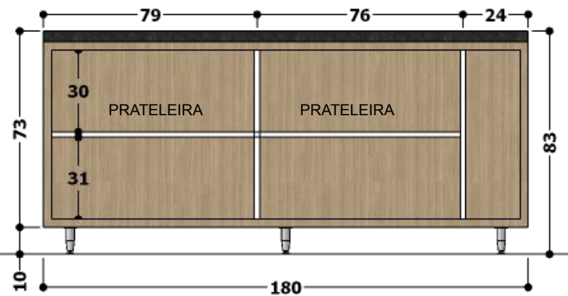
VISTA INTERNA – BALCÃO COM PORTAS.
