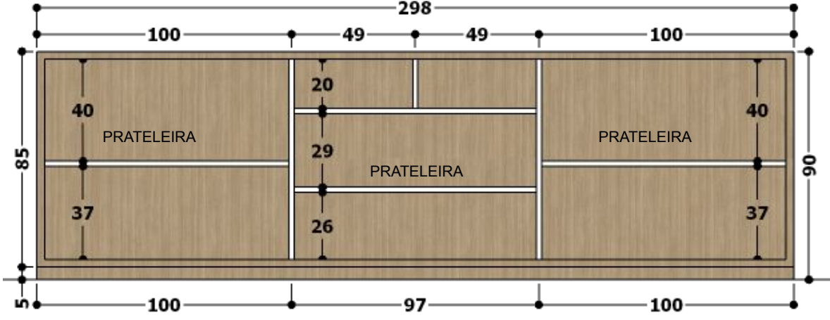
VISTA FRONTAL – BALCÃO COM PORTAS.
