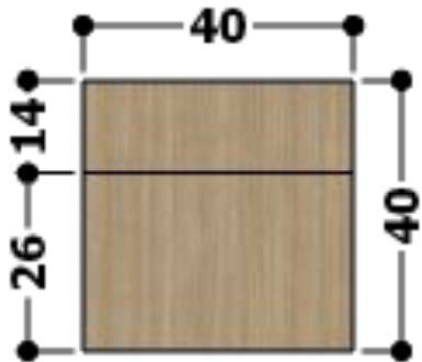
VISTA FRONTAL – MESA DE APOIO COM PORTA E RODÍZIO
