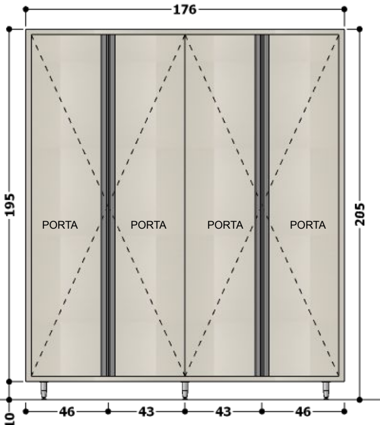
VISTA FRONTAL – ARMÁRIO COM PORTAS.
