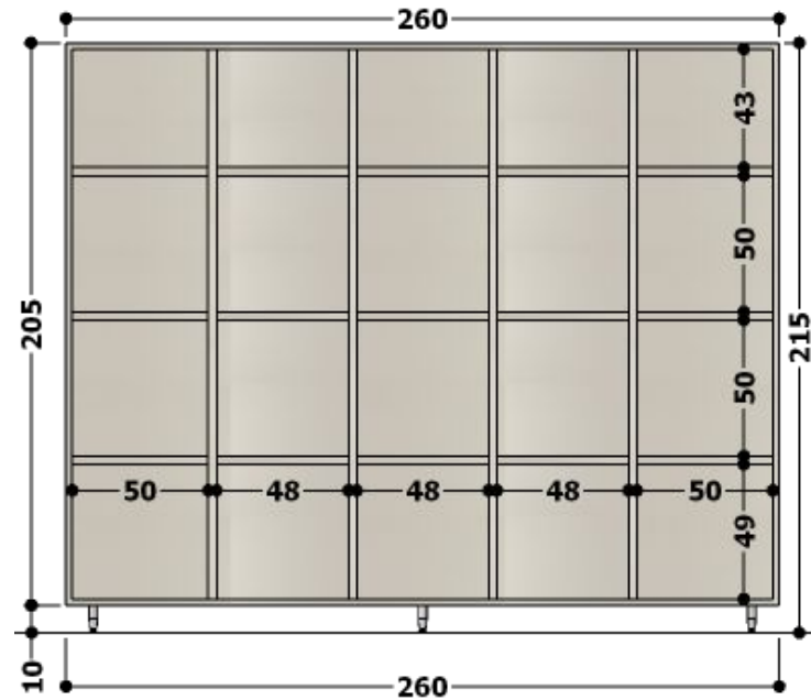
VISTA FRONTAL – ARMÁRIO DE NICHOS.
