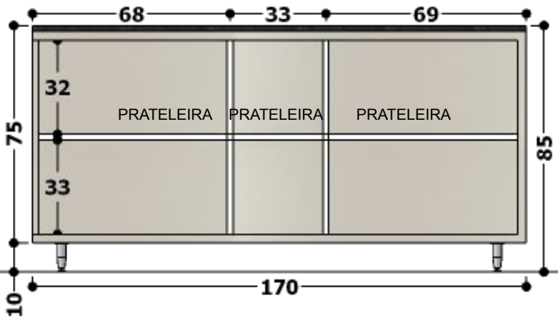
VISTA INTERNA – GABINETE COM PORTAS.
