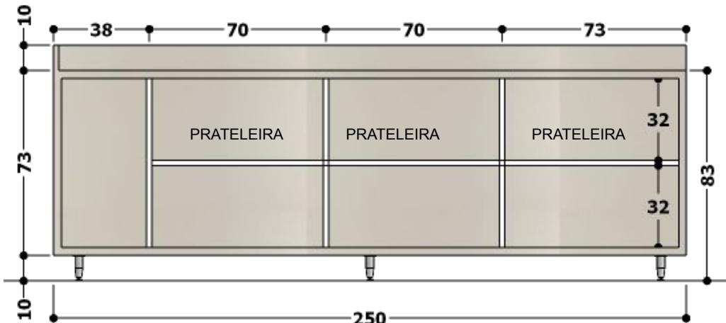
VISTA INTERNO – BALCÃO COM PORTAS.
