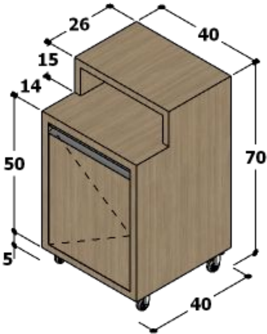
* MÓVEL EM MDF CARVALHO DIAN - DURATEX, COM PUXADORES EM PERFIL G EM ALUMÍNIO, BASE/ PÉ EM RODÍZIO.
