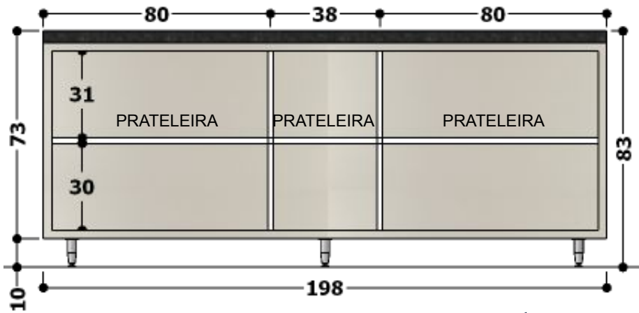
VISTA INTERNA – GABINETE COM PORTAS.
