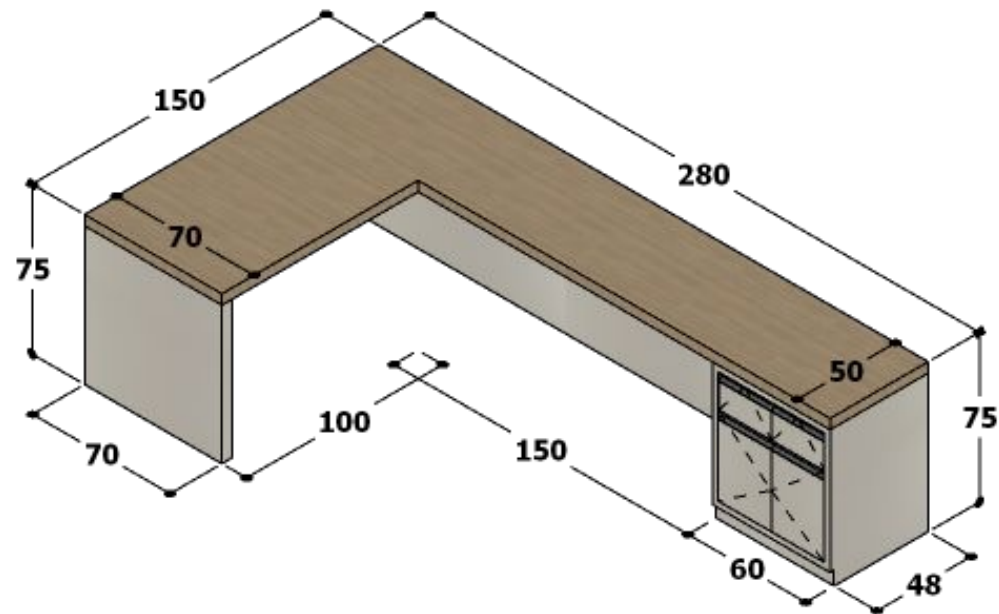
VISTA PERSPECTIVADA – MESA EM L COM GAVETAS.
