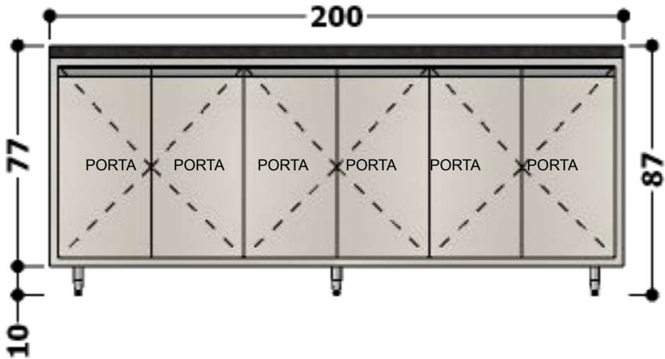
VISTA FRONTAL – GABINETE COM PORTAS.
