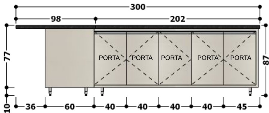
VISTA FRONTAL – GABINETE EM L.
