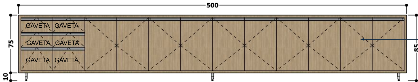
VISTA FRONTAL – ARMÁRIO BAIXO COM PORTAS.
