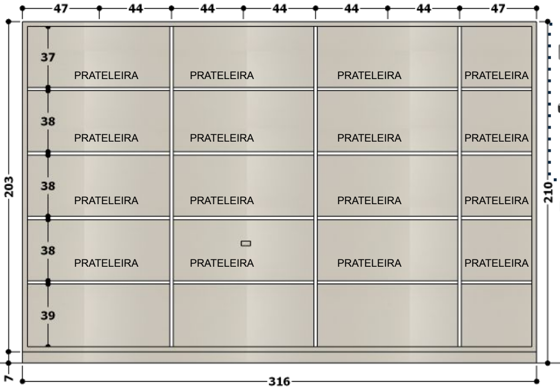
VISTA INTERNA – ARMÁRIO COM PORTAS.
