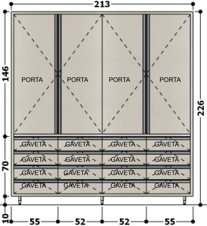
VISTA FRONTAL – ARMÁRIO COM PORTAS E GAVETAS.
